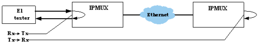
Fig 3.2.2-3 E1 loop back
